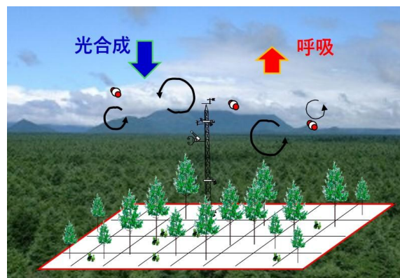
図 2 \text{CO}_2 の吸収・放出量の観測手法の概略図 中央の気象観測タワーを用いて、大気中の \text{CO}_2 の流れをリアルタイムにモニターすることで、 \text{CO}_2 の吸収・放出量を 30 分毎に連続測定できる。
