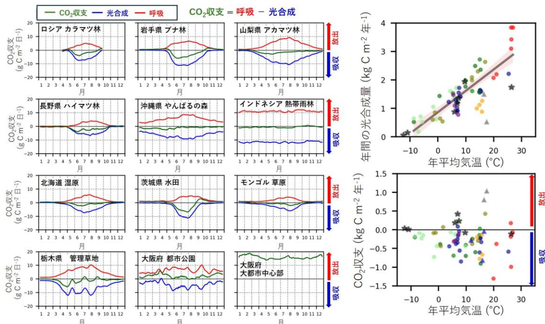
図 3 いくつかの生態系・都市を対象とした \text{CO}_2 収支の平均的な季節変化パターン \text{CO}_2 収支および年間の光合成量を示したグラフにおけるシンボルの違いは、異なる生態系タイプを示す。
