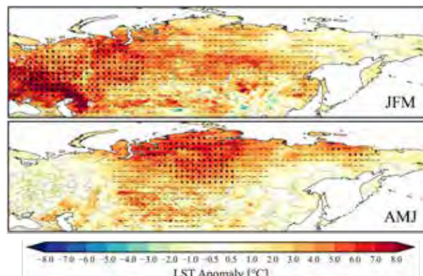
2020年冬～春のシベリアの異常高温のモニタリング（図は衛星観測による地表面温度の異常値を示す） Land surface temperature anomalies across Siberia during winter to spring in 2020.
