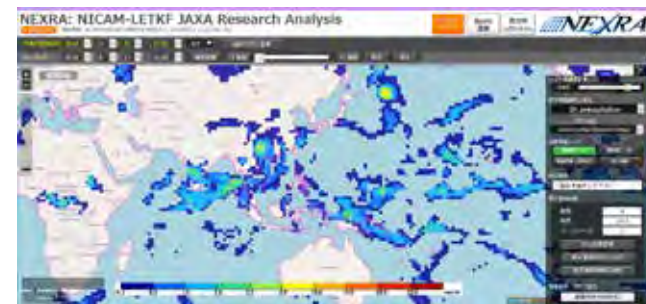
JAXA のスパコンで準実時間運用されている全球大気データ同化システム NEXRA The near-real-time global atmospheric data assimilation system NEXRA running on the JAXA's supercomputing system
