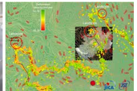
マレー半島にて地殻変動地域（土砂崩れなど）の 3 次元マッピング (JICA-JST 事業) 3D mapping of land deformed area (landslide etc) at Malay Peninsula under JICA-JST Project
